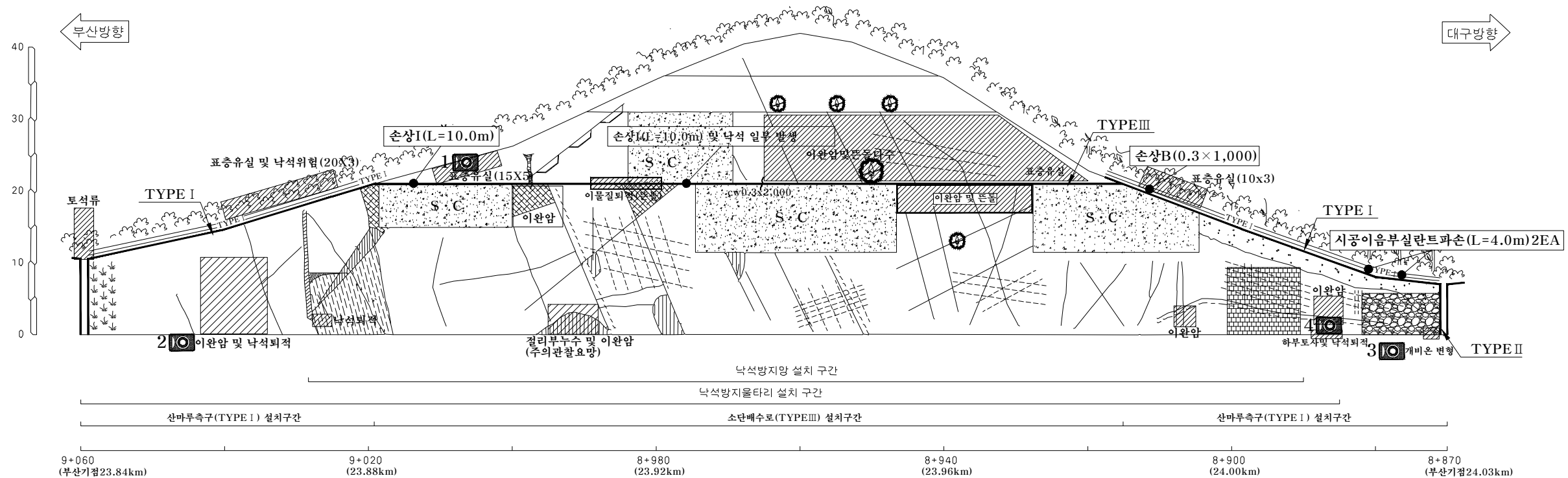
부산절토36/부산기점 23.84~24.03km (9공구 STA.8+870~9+060)
